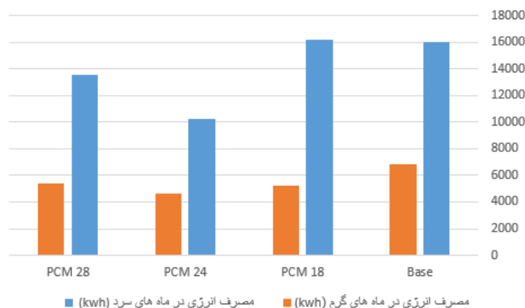
شکل ۳: میزان مصرف انرژی در ماه‌های گرم و ماه‌های سرد در دو وضعیت پایه و PCM در جدارهای خارجی - سالانه Fig 3: The amount of energy consumption in hot and cold months in both basic and PCM conditions in external walls on an annual basis
