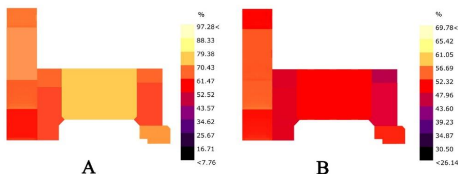
شکل ۹: نتایج شاخص ATPC برای محیط حوضخانه: (A) با حضور آب؛ (B) بدون حضور آب Fig. 9: Pool house ATPC diagram: (A) presence of water; (B) absence of water
