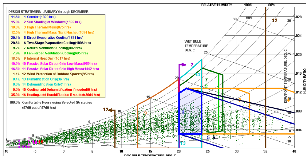
شکل ۲. نمودار سایکرومتریک شهر تبریز و حوزه آسایش حرارتی در آن (برگرفته از ورژن ۱۰ نرم‌افزار کلایمیت کانسلنت (Climateconsultant)
