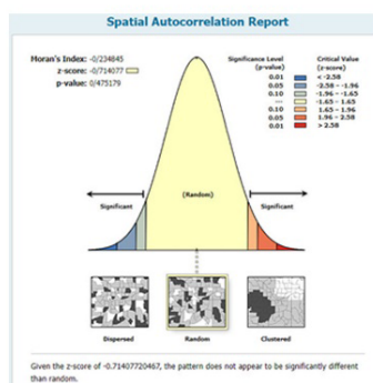
شاخص‌های خود همبستگی فضایی محلات "نسبتاً کم برخوردار" Spatial autocorrelation index for relatively poor districts
