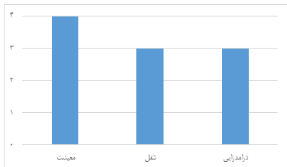
نمودار ۱۰: مؤلفه‌های اقتصادی سبک زندگی متأثر از معماری از نگاه پژوهش‌های صورت پذیرفته
