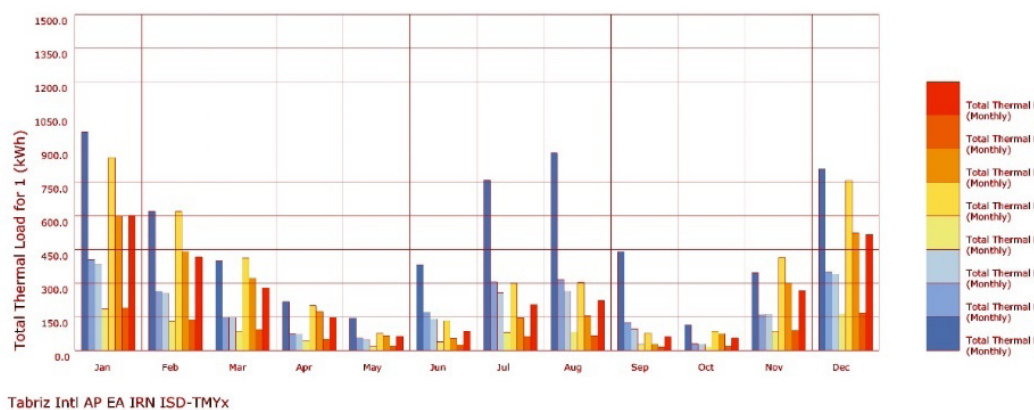
شکل ۶: میزان مصرف انرژی به تفکیک فضاها در وضعیت پایه در طی سال Fig 6: The amount of energy consumption by different spaces in the basic state during the year
