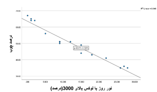
شکل ۱۰. نمودار همبستگی درصد چوب با میزان درخشندگی Figure 10. Correlation Chart of Wood Percentage with Radiance
