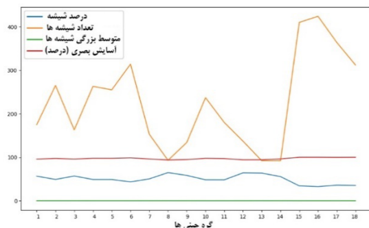
شکل ۱۷. نمودار ارتباط درصد شیشه، تعداد شیشه و میانگین بزرگی تکه شیشه‌ها با آسایش بصری
